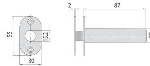
Кабелепроходы 06.515.00.0 06.515.15
