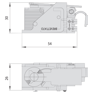
Сменные катушки регулируемые 07.120.00.2 (12V) 07.120.01.2 (24V)
